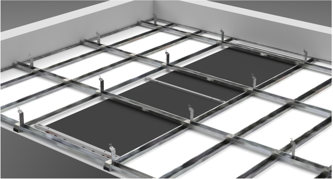
Paneeli asennettuna.
